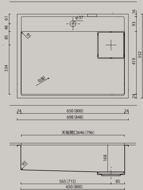
標準仕様排水口 (対応排水部品セット：A)
