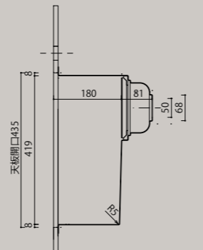
一体仕様排水口 (対応排水部品セット：B)
